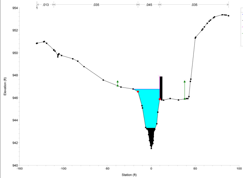
SECTION A-B
